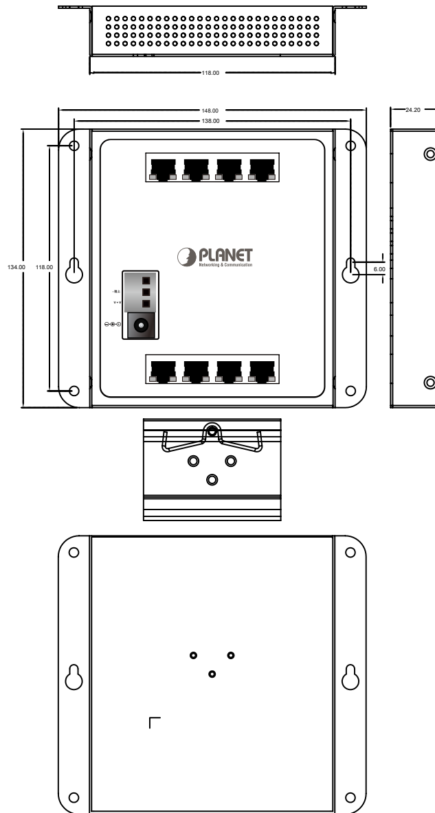
寸法 (単位mm)
